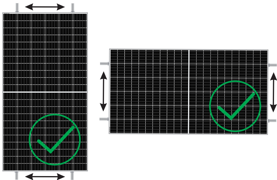
Fixação do módulo pelo lado menor
