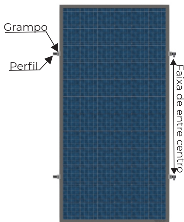
Instalação do módulo em posição retrato
