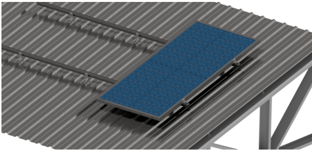
Instalação do módulo em posição retrato
