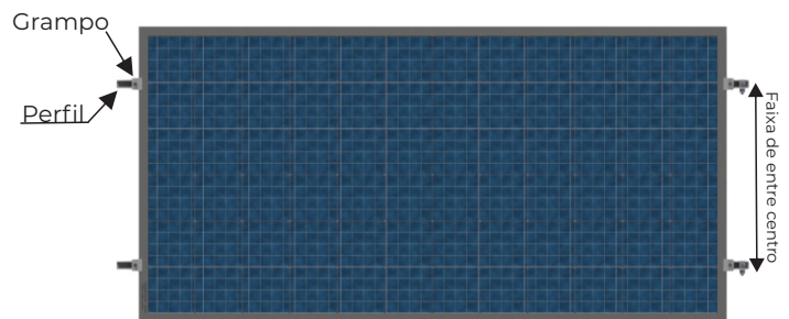
Instalação do módulo em posição paisagem
